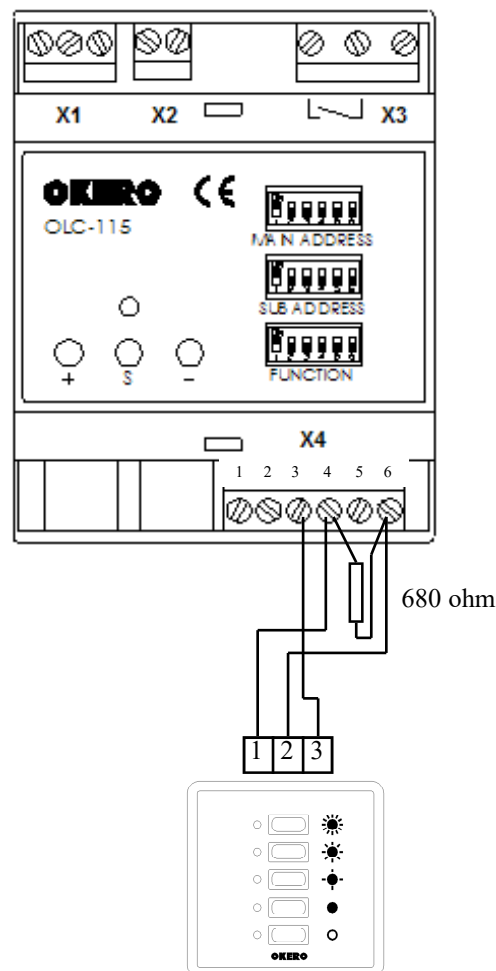
Figur 3. Inkoppling av DML panel.
