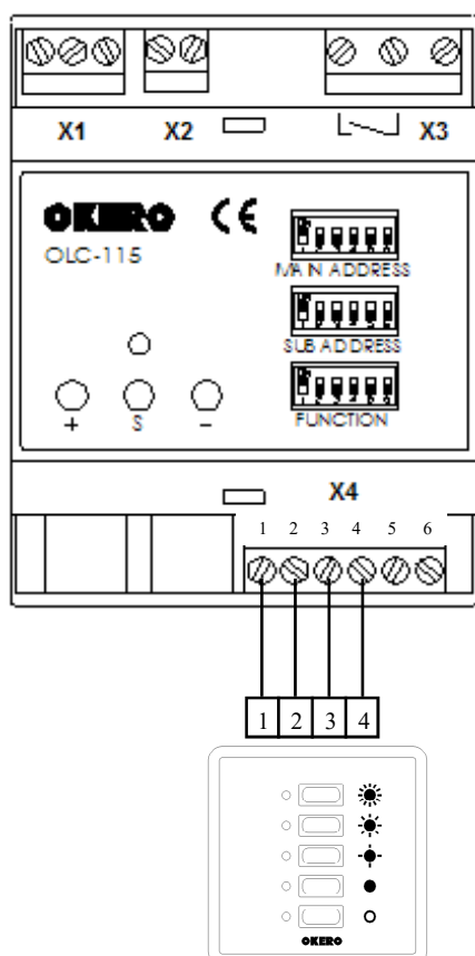
Figur 2. Inkoppling av OLC panel
